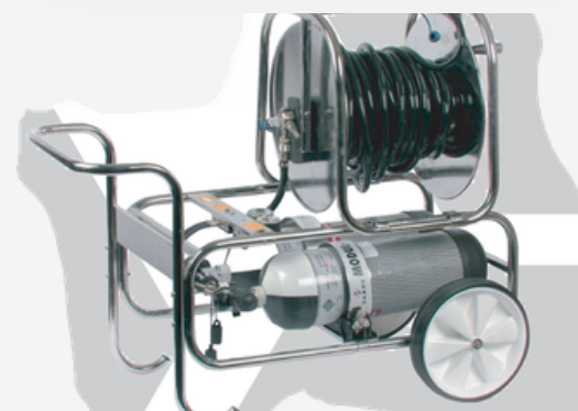
▲ 氣樽及氣體
